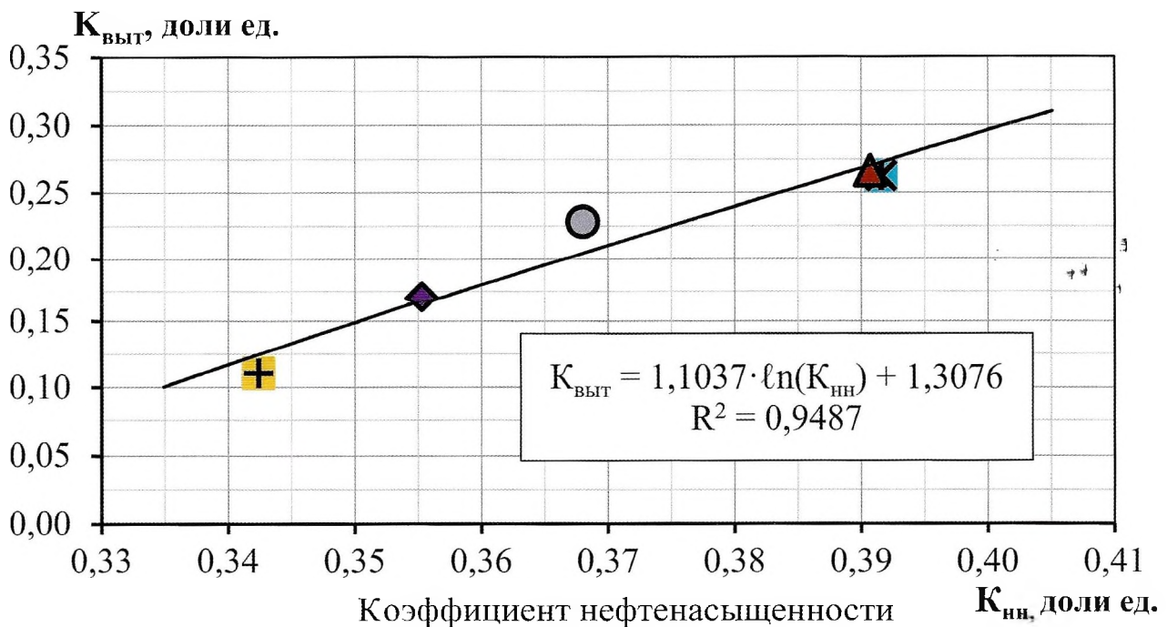
Рис. 7. Обобщённая (усреднённая по данным 44 опытов) зависимость коэффициента вытеснения нефти водой от начальной нефтенасыщенности образцов керн по УНПК Приобского месторождения (южная часть)
