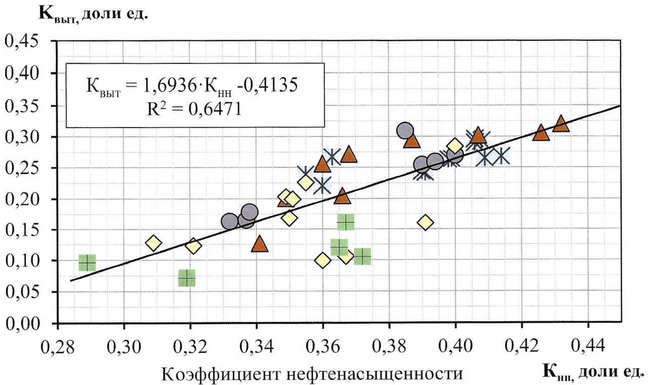
Рис. 6. Сопоставление коэффициентов вытеснения нефти водой и начальной нефтенасыщенности образцов керн из УНПК Приобского месторождения – по первичным данным 44 опытов
