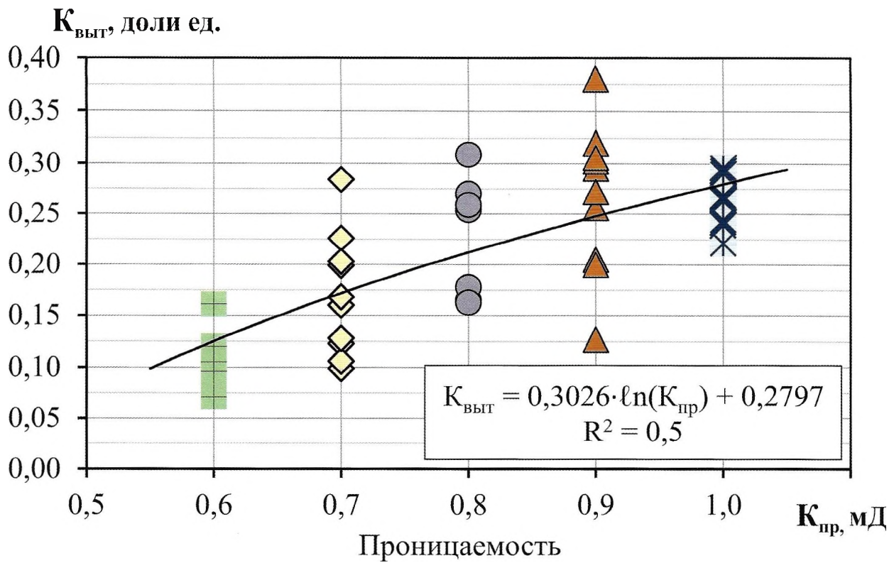
Рис. 4. Сопоставление коэффициента вытеснения нефти водой и абсолютной проницаемости образцов керна по УНПК Приобского месторождения (южная часть) – по первичным данным 44 опытов
