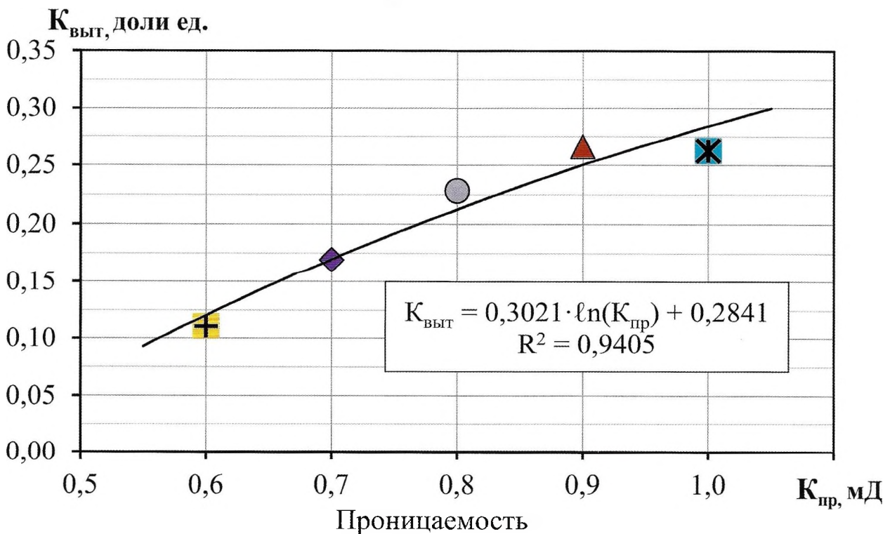
Рис. 5. Обобщённая (усреднённая по данным 44 опытов) зависимость коэффициента вытеснения нефти водой от абсолютной проницаемости образцов керна из УНПК пластов АС 9,12 Приобского месторождения (южная часть)
