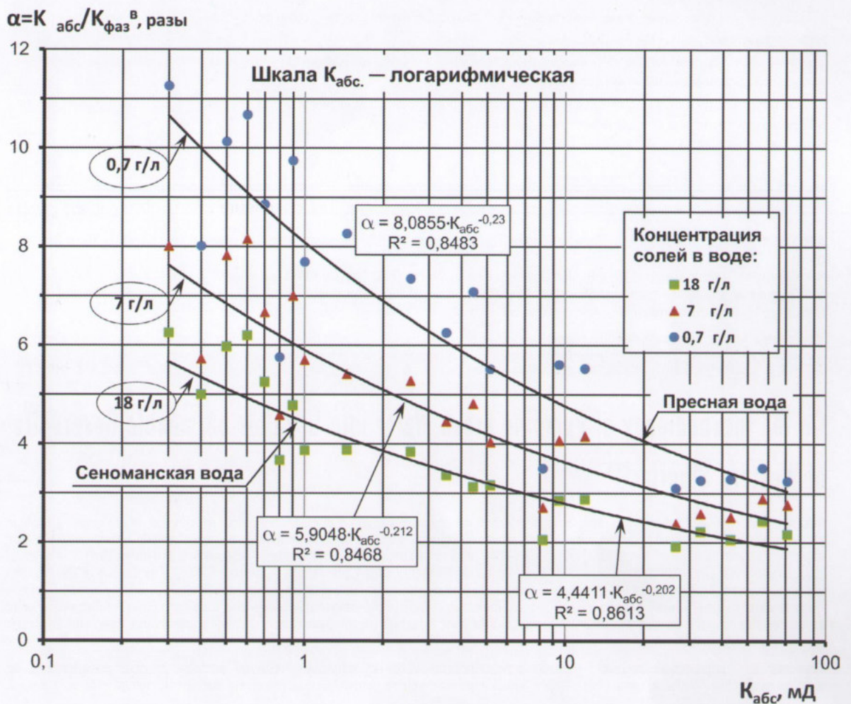
Рис. 2. Зависимости степени снижения K_{фаз}^в (разы) на керне от абсолютной проницаемости K_{абс} образцов (в логарифмическом масштабе) и минерализации прокачиваемой воды
